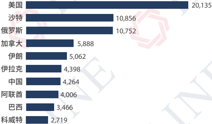
图2：2024年全球石油生产量分布图
