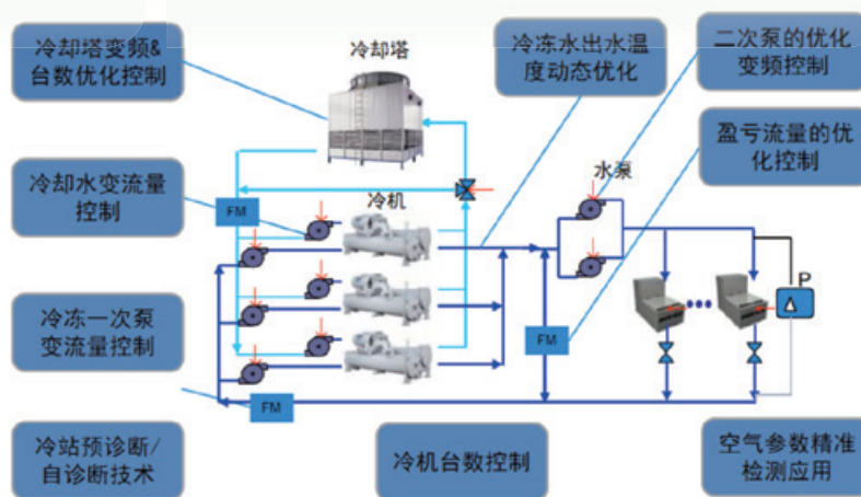
▲ 冷冻机 CCN 群控系统优化
